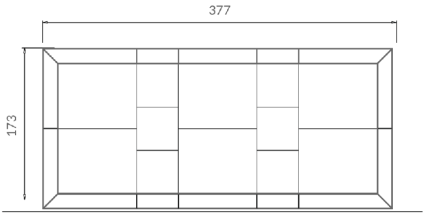
INTRECCIO – cm 377,3x6,5xH173
