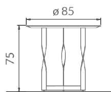
ø 85xH75
