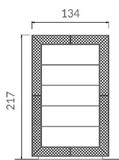
cm 134x40x217
