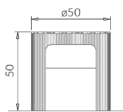
cm ø50xH50
