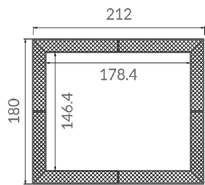
cm 212x13xH180
