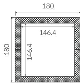
cm 180x13xH180
