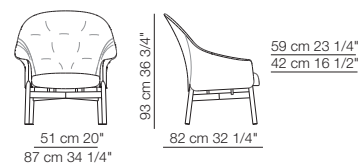
Poltrona con schienale alto versione trapunta morbida Armchair with high backrest version with soft quilt
