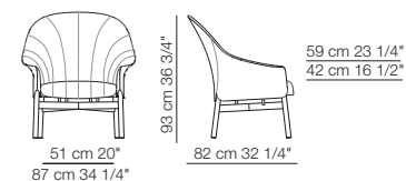
Poltrona con schienale alto versione trapunta rigata Armchair with high backrest version with striped quilt
