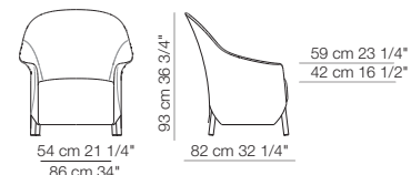
Poltrona con schienale alto e gonnella Armchair with high backrest and skirt
