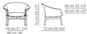
Poltrona con schienale basso Armchair with low backrest
