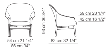
Poltrona con schienale alto Armchair with high backrest
