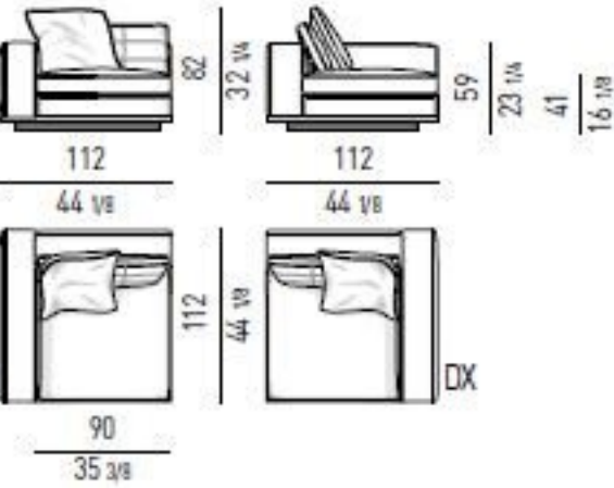
ELEMENTO TERMINALE CM 112 - BRACCIOLO ALTO ELEMENT WITH 1 ARMREST CM 112 - HIGH ARMREST
