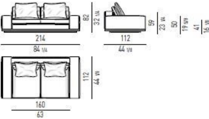
DIVANO CM 214 - BRACCIOLO BASSO SOFA CM 214 - LOW ARMREST
