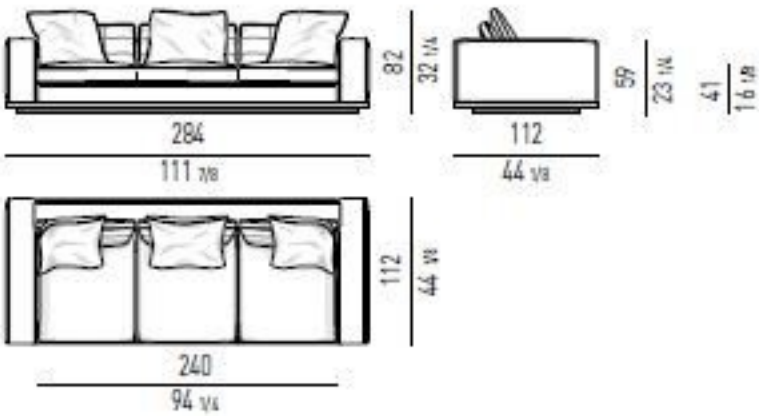
DIVANO CM 284 - BRACCIOLO ALTO SOFA CM 284 - HIGH ARMREST
