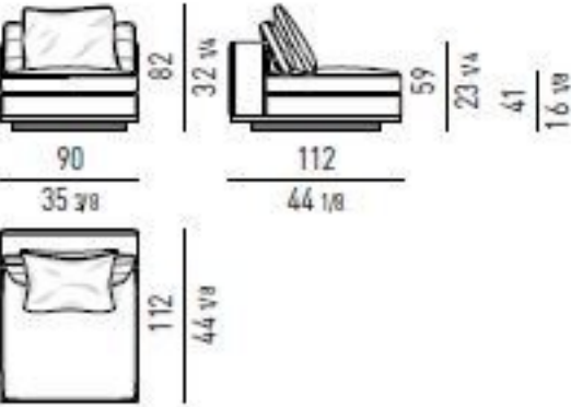
ELEMENTO CENTRALE CM 90 CENTRAL ELEMENT CM 90
