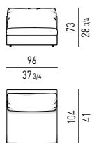
ELEMENTO CENTRALE CM 96 CENTRAL ELEMENT CM 96
