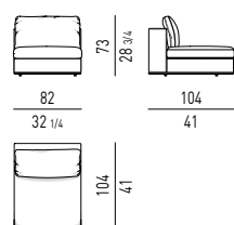
SOFÀ SENZA BRACCIOLO CM 82 SOFÀ WITHOUT ARMRESTS CM 82
