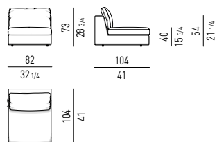
ELEMENTO CENTRALE CM 82 CENTRAL ELEMENT CM 82
