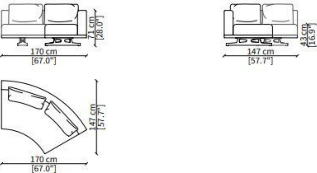
Elemento 60° / Element 60°
