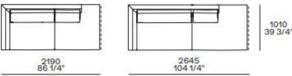
Terminale penisola sx-dx con bracciolo alto Lt-rt peninsula end unit with high arm
