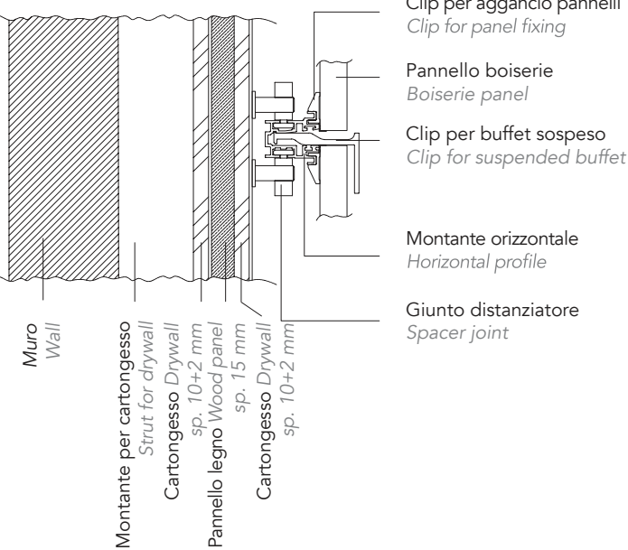
b) Aggancio su cartongesso Drywall mounting
