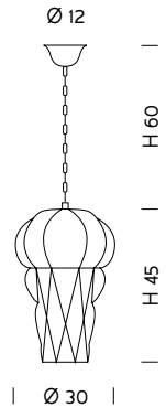
1443/30 1 x MAX 70W E27
