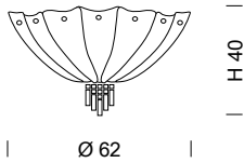
420/62 4 x MAX 70W E27 + 1 x MAX 50W GU10
