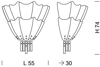
421/A5 5 x MAX 70W E27
