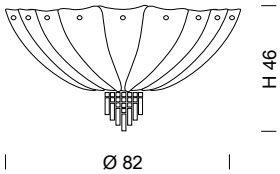
420/82 6 x MAX 70W E27 + 1 x MAX 50W GU10
