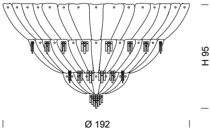
420/192 40 x MAX 70W E27 + 1 x MAX 42W E14
