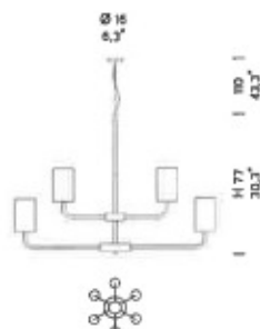
2120/12+6 18 x MAX 42W E14 (E)
