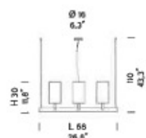
2120/9+3 12 x MAX 42W E14 (E)
