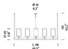
2120/12+6 18 x MAX 42W E14 (E)
