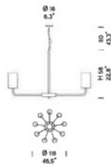
2120/12 12 x MAX 42W E14 (E)
