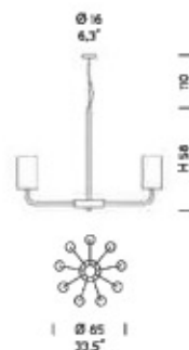
2120/9 9 x MAX 42W E14 (E)
