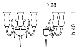
1022/A3 3 x MAX 42W E14
