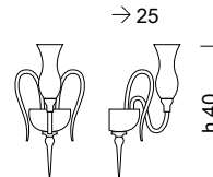
1022/A1 1 x MAX 42W E14
