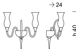
1022/A2 2 x MAX 42W E14
