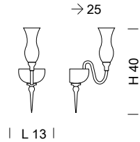
1020/A1 1 x MAX 42W E14
