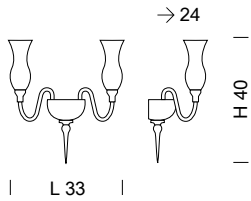
1020/A2 2 x MAX 42W E14
