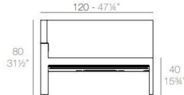
FRAME Sofá Módulo Derecho FRAME Sectional Sofa Right
