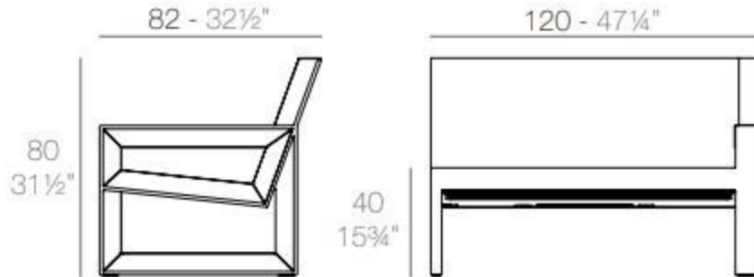
FRAME Sofá Módulo Izquierdo FRAME Sectional Sofa Left
