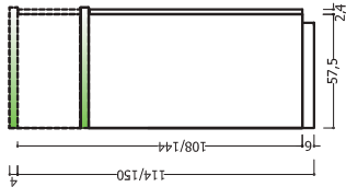
COLONNE H 114 - 150 COLUMNS H 114 - 150
