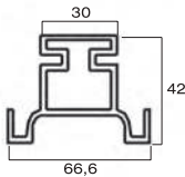
Sezione gola tipo "D" Type "D" finger rail section
