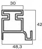
Sezione gola tipo "C" Type "C" finger rail section
