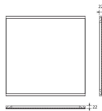
anta MODULO CENTRALE door CENTRAL MODULE
