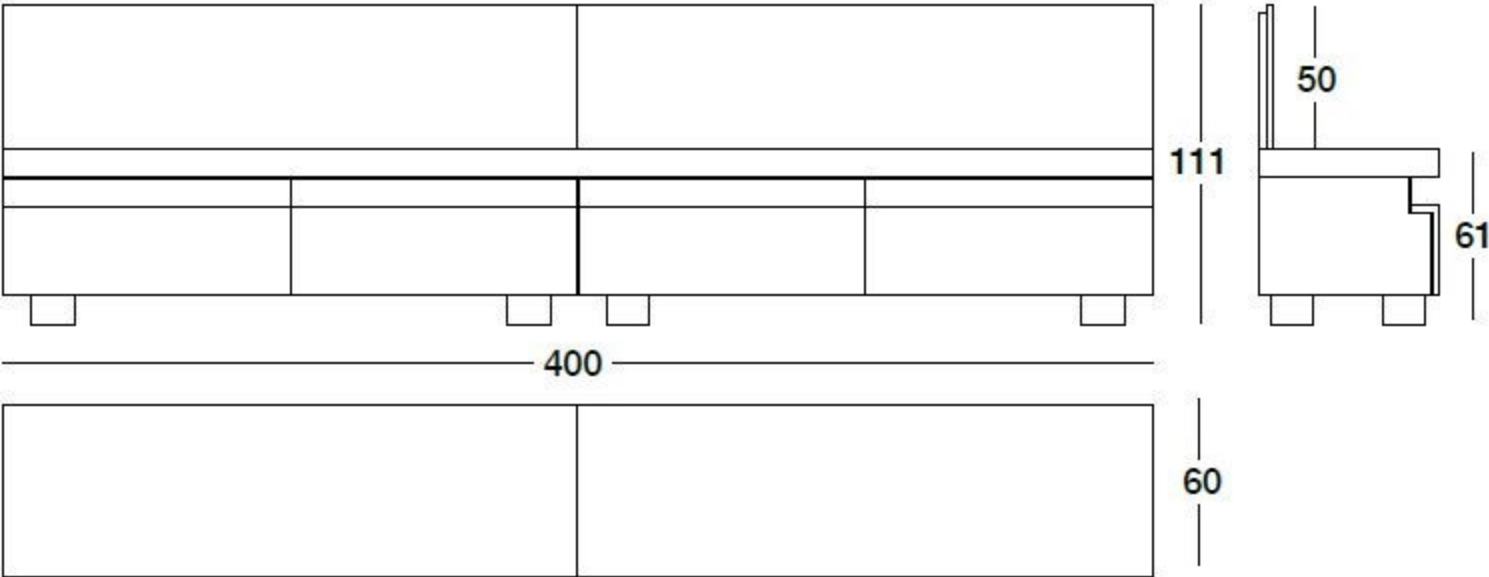
Composizione 4 cassettoni con o senza schienale / Composition of 4 large drawers with or without back panel / Композиция из 4 больших ящиков с задней панелью или без нее
