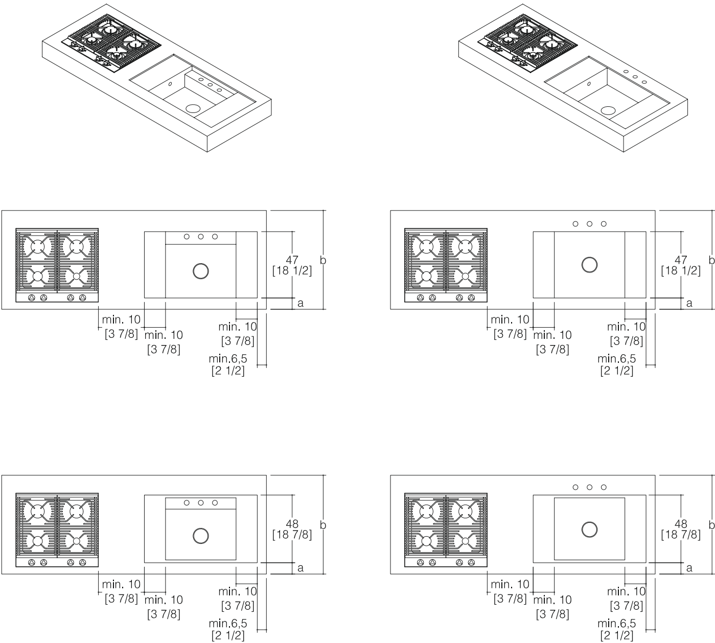
MODULARITÀ vista in pianta e assonometrica MODULARITY plan view and assonometric view
