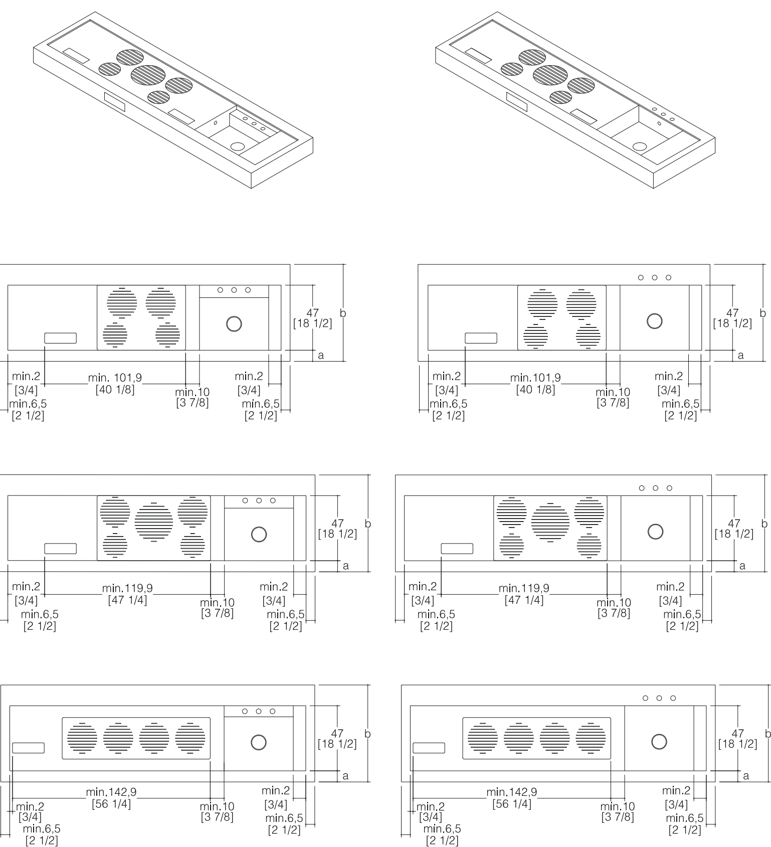
MODULARITÀ vista in pianta e assonometrica MODULARITY plan view and assonometric view
