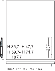
PENSILE WALL UNIT
