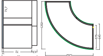
ISOLA CIRCOLARE TIPO "D" 1202 X 1224 ROUND ISLAND UNIT TYPE "D"
