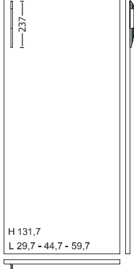
COLONNA 1 ANTA COLUMN DOOR
