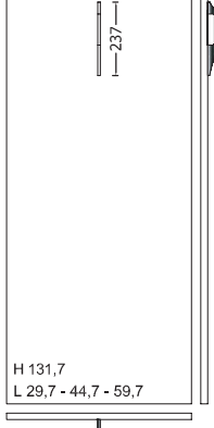
COLONNA ANTA CESTELLO ESTRAIBILE COLUMN PULL-OUT BASKET DRAWER DOOR
