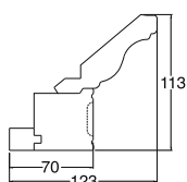
cornice Royal con fresate N.B.: per le finiture vedi colori ante grooved Royal top cornice Note: for the finishes see door colours
