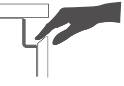
Preso Inclinata 40° 40° angled grip edge
